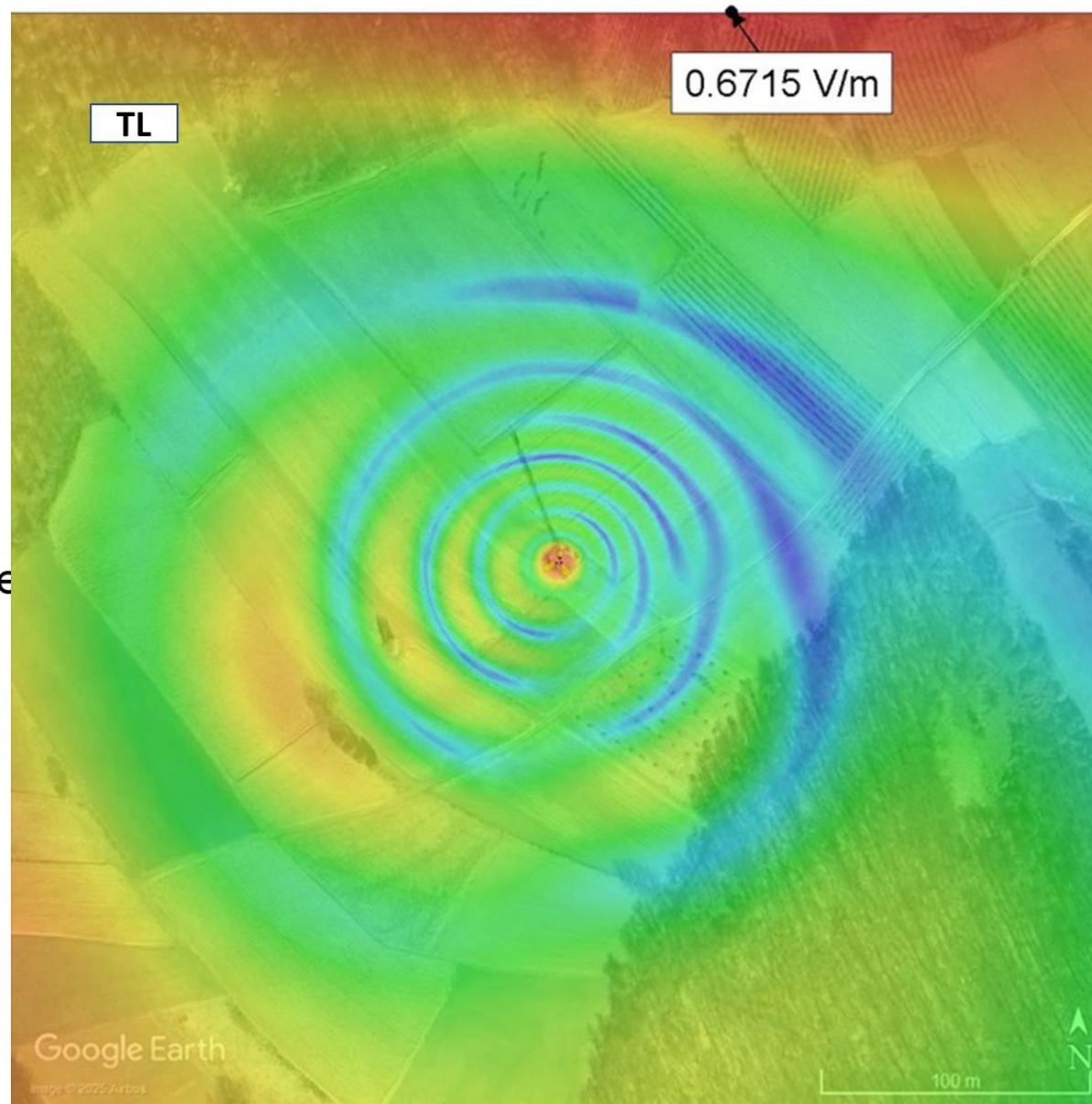
Слика 4.4. Јачина електричног поља на тлу, на јавном подручју, када радио-систем LTE700 оператора Cetin ради максималним капацитетом
