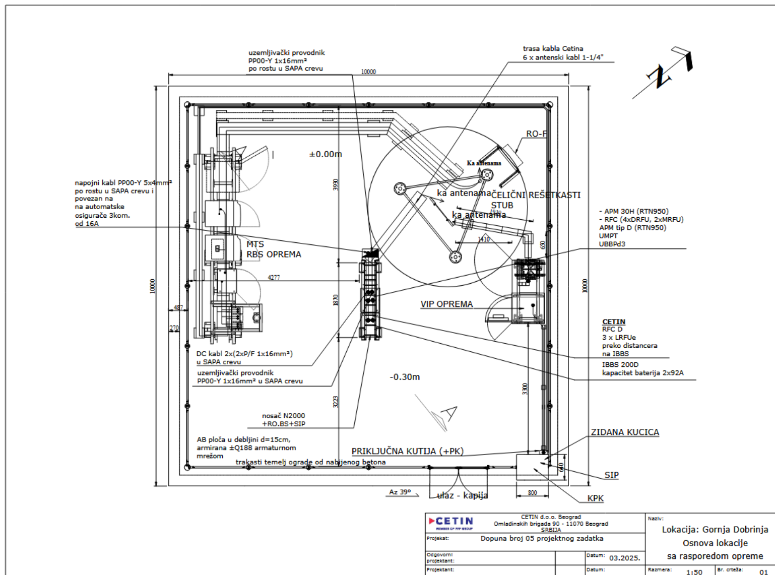
Слика 8.1. Идејно решење – Основа локације са распоредом опреме
