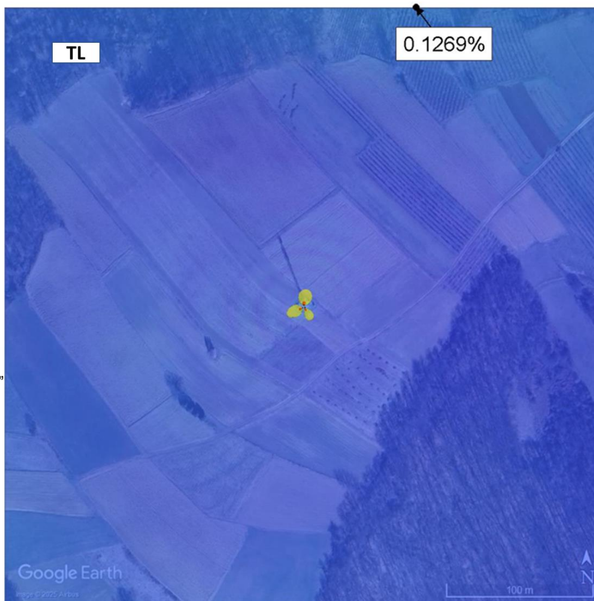
Слика 4.7. Фактор изложености на тлу, на јавном подручју, када сви радио-системи оператора Cetin раде максималним капацитетом
