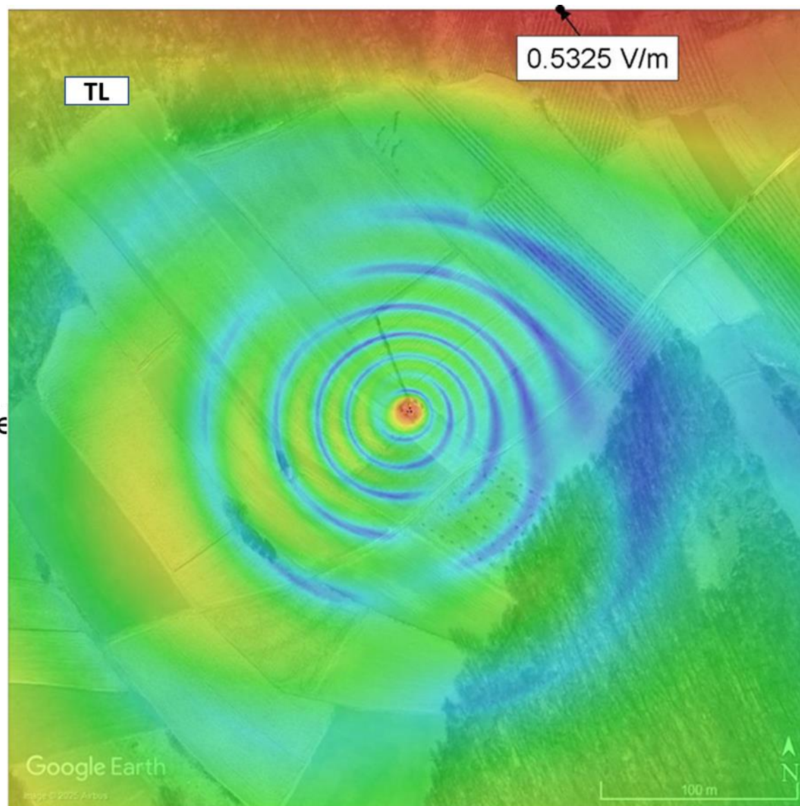
Слика 4.3. Јачина електричног поља на тлу, на јавном подручју, када радио-систем UMTS900 оператора Cetin ради максималним капацитетом
