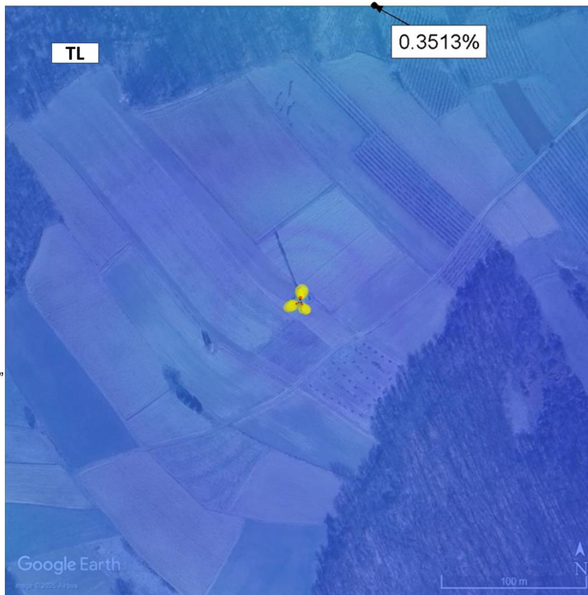
Слика 4.8. Фактор изложености на тлу, на јавном подручју, када сви радио-системи свих оператора раде максималним капацитетом
