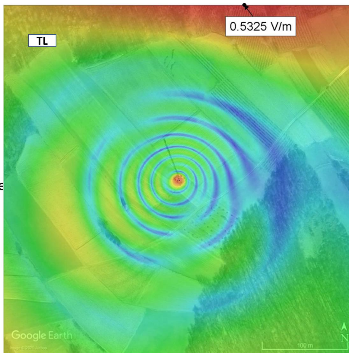
Слика 4.2. Јачина електричног поља на тлу, на јавном подручју, када радио-систем GSM900 оператора Cetin ради максималним капацитетом
