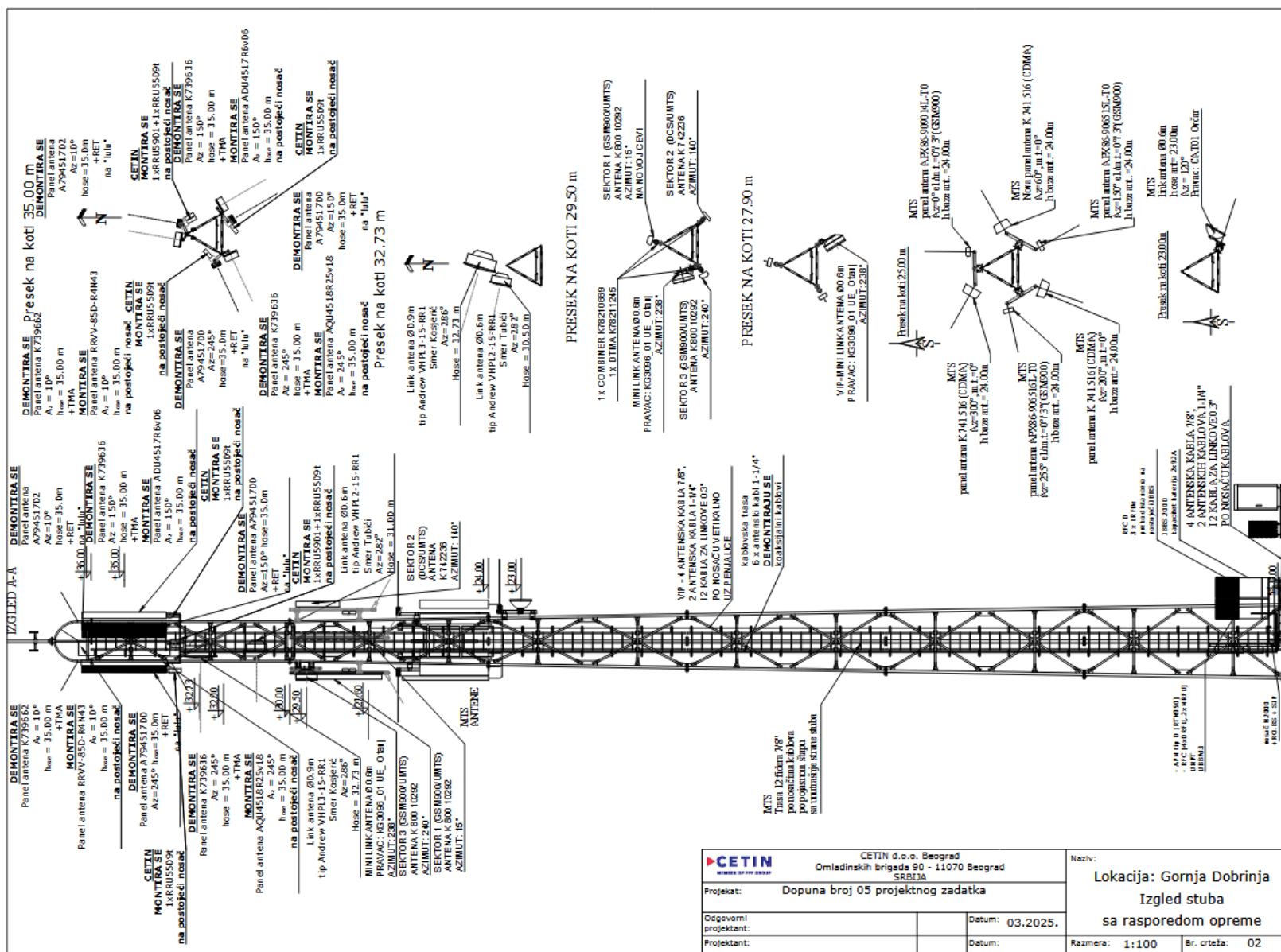
Слика 8.2. Идејно решење – Изглед стуба са распоредом опреме
