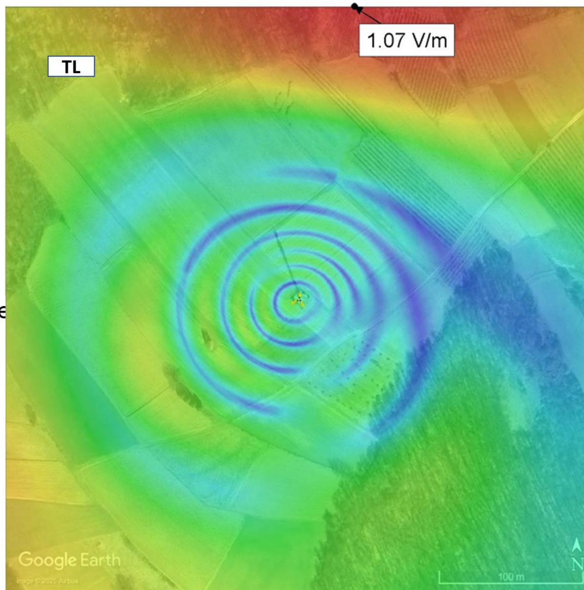
Слика 4.5. Јачина електричног поља на тлу, на јавном подручју, када радио-систем LTE800 оператора Cetin ради максималним капацитетом
